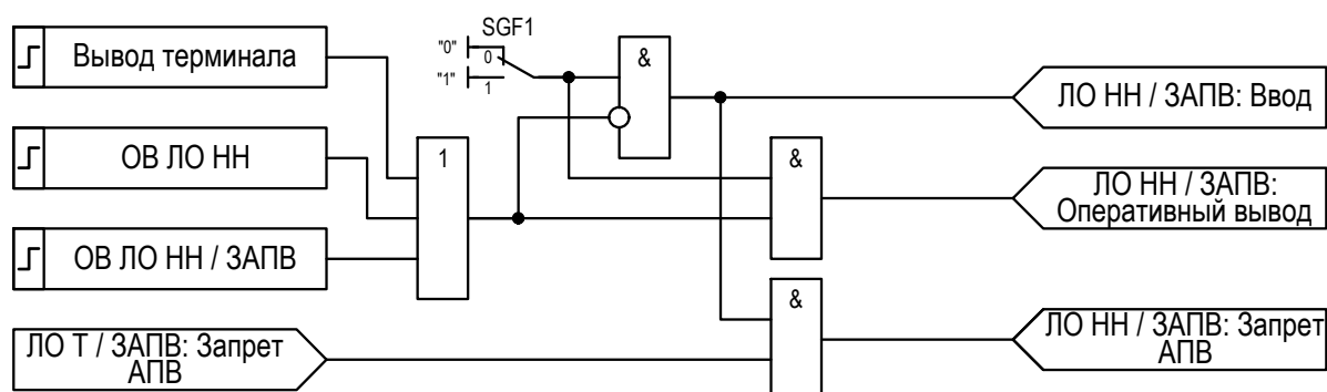
Рисунок 2.24 – Функциональная схема «Запрет АПВ»
