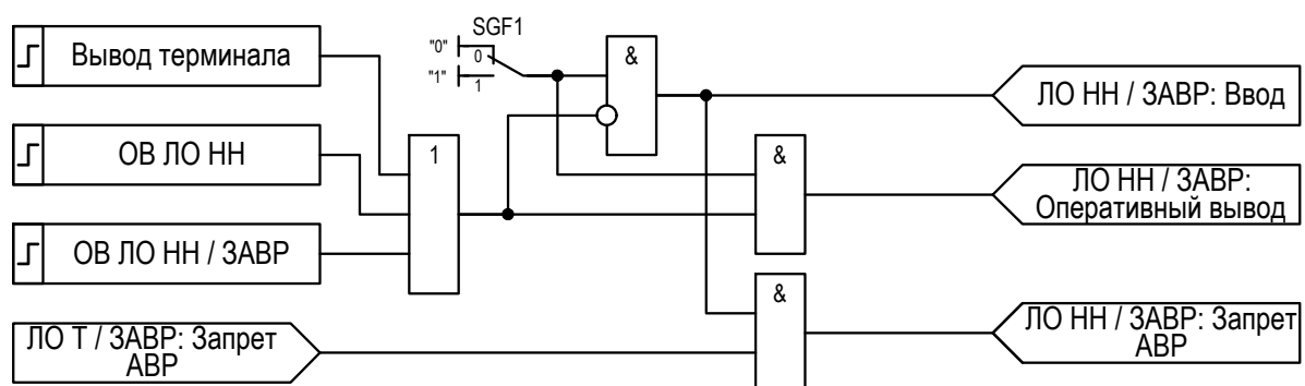
Рисунок 2.25 – Функциональная схема «Запрет АВР»
